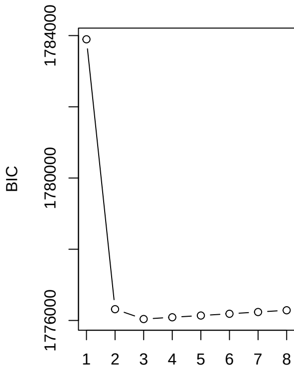
BIC
